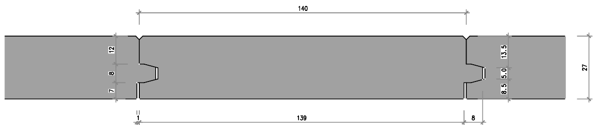
Nr. 4663-M2k-01 Spitzkamm 27/140 mm, Fase 1.5 mm
