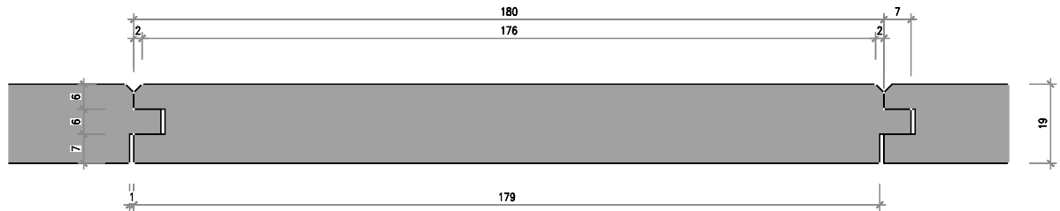
Nr. 1103-2k-01 Fastäfer 19/180 mm, Fase 1.5 mm
