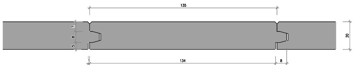
Nr. 4663-M2k-01 Spitzkamm 20/135 mm, Fase 1.5 mm
