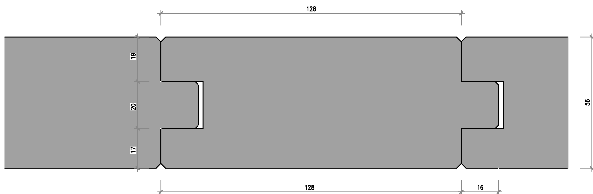
Nr. 4143-S4k-02 Strickwand 56/128 mm, Fase 4-seitig 2 mm
