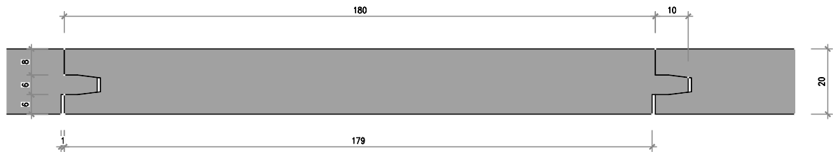
Nr. 4155-0k-00 Spezial N+K, Kamm 10 mm lang konisch
