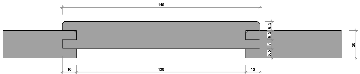
Nr. 6303-2k-01 Hoch-Tiefschalung 20/140 mm
