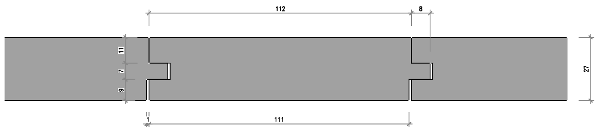
Nr. 4145-M Bodenriemen 27/112 mm
