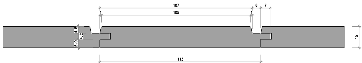
Nr. 2105-06-00 Sichtnuttäfer 15/113 mm, Nut 6 mm
