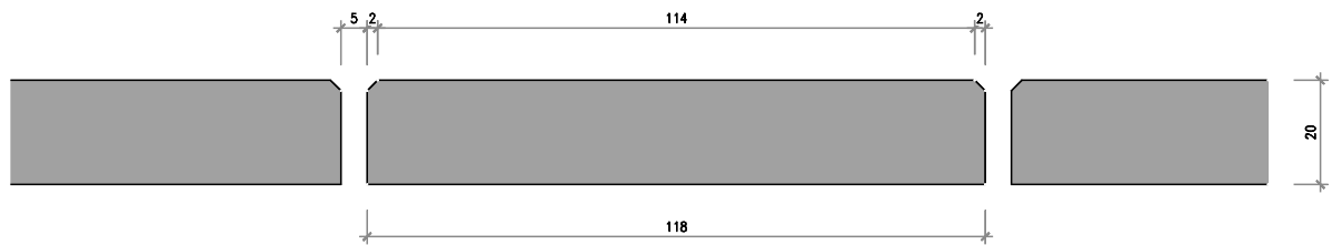
Nr. 6103-2k-02 Akustiktäfer 20/118 mm, Fase 2 mm
