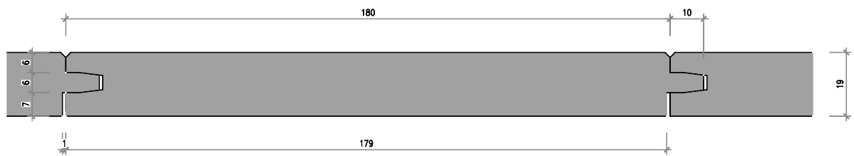
Nr. 4153-2k-01 Spezial Fastäfer 19/180 mm, Fase 1.5 mm
