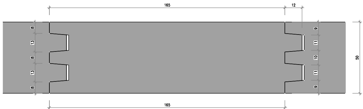
Nr. 4755-L Doppel-Nut und Kamm 50/165 mm
