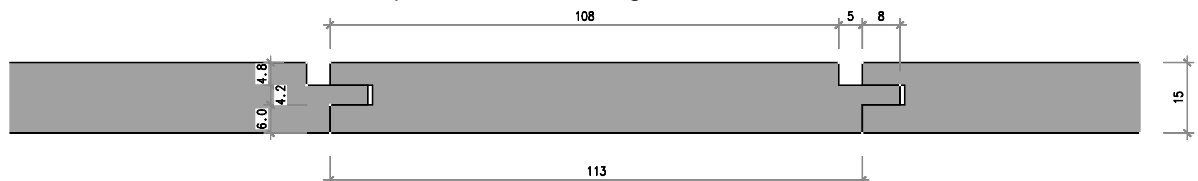
Nr. 2205-05-00 Spezial Sichtnuttäfer gerade 15/113 mm, Nut 5 mm
