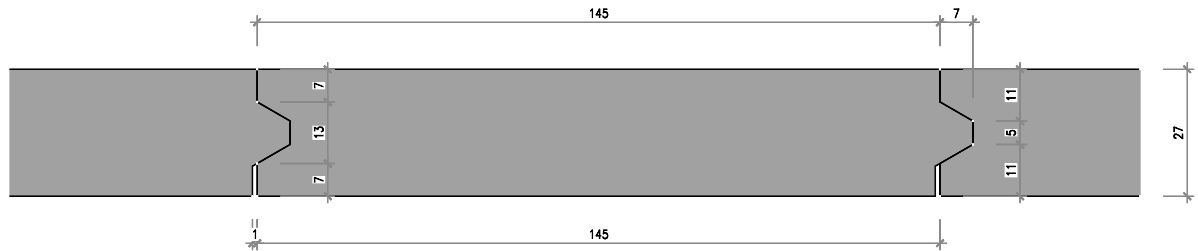
Nr. 4665-L Blindschalung 27/145 mm, Kamm 30°
