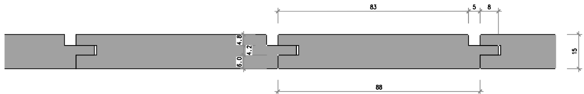
Nr. 2205-05-00 Spezial Sichtnuttäfer gerade 15/88 mm, Nut 5 mm
