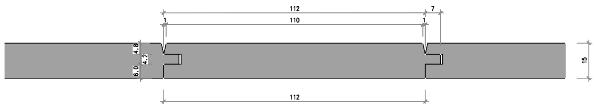
Nr. 1205-02-00 Steilfastäfer 15/112 mm
