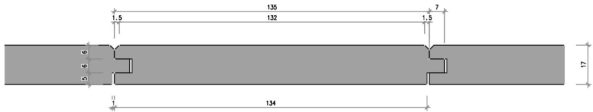
Nr. 1103-2k-01 Fastäfer 17/135 mm, Fase 1.5 mm
