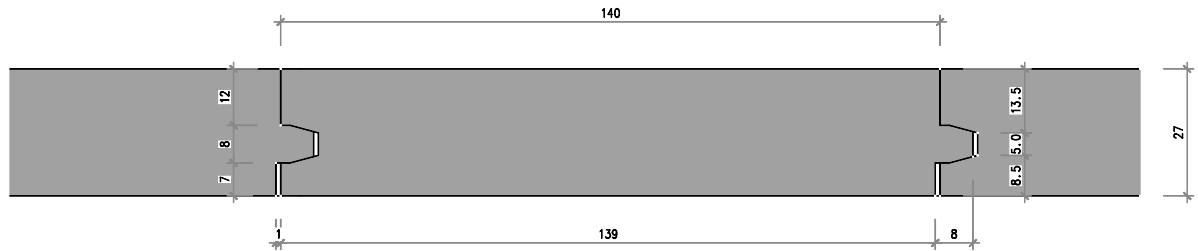
Nr. 4665-M Spitzkamm 27/140 mm
