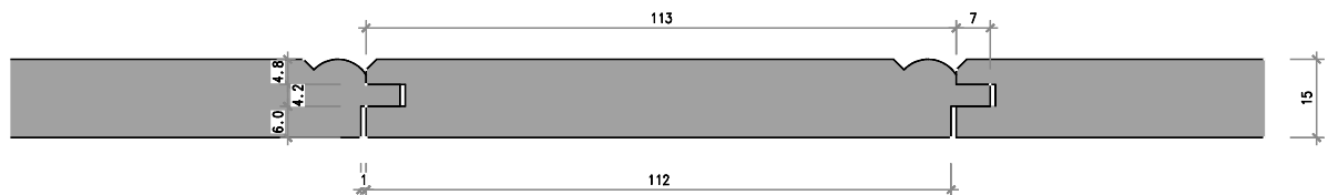
Nr. 5203-12-02 Krallentäfer 15/113 mm
