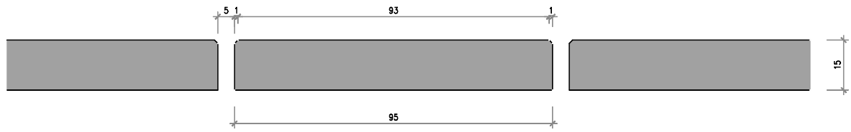
Nr. 6103-2k-01 Akustiktäfer 15/95 mm, Fase 1 mm
