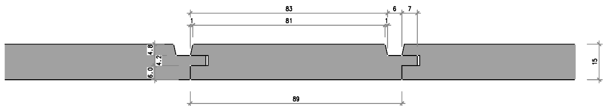
Nr. 2105-06-00 Sichtnuttäfer 15/89 mm, Nut 6 mm
