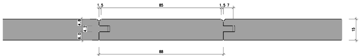
Nr. 1103-2k-01 Fastäfer 15/88 mm, Fase 1.5 mm
